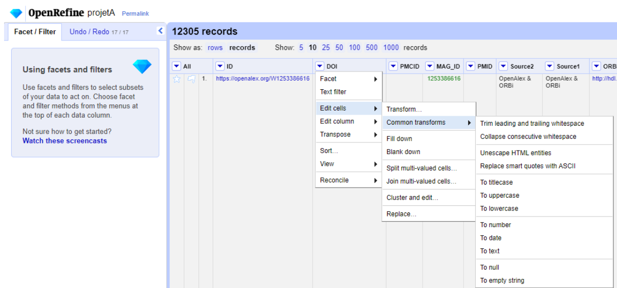
Fig.11 : Marche à suivre de sélection pour appliquer les transformations de données au sein d’une colonne.
